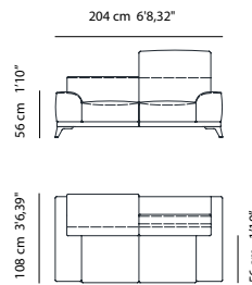
Sofá 3 plazas reducido_ Ref. 106250
